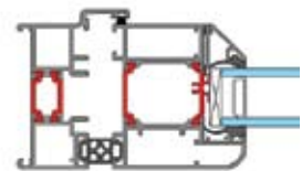
Jamb Detail
